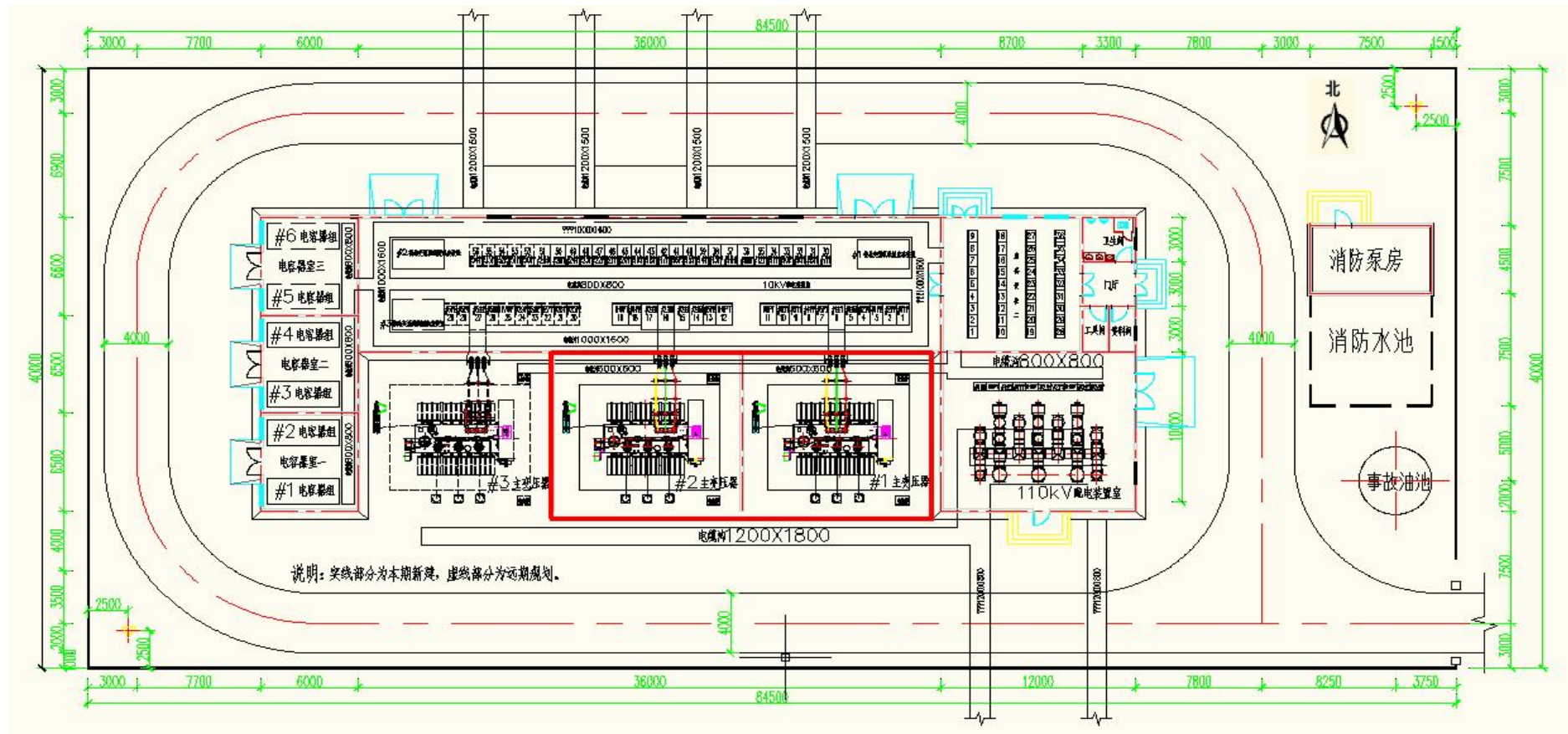
附图 3 养马庄 110kV 变电站电气平面布置图
