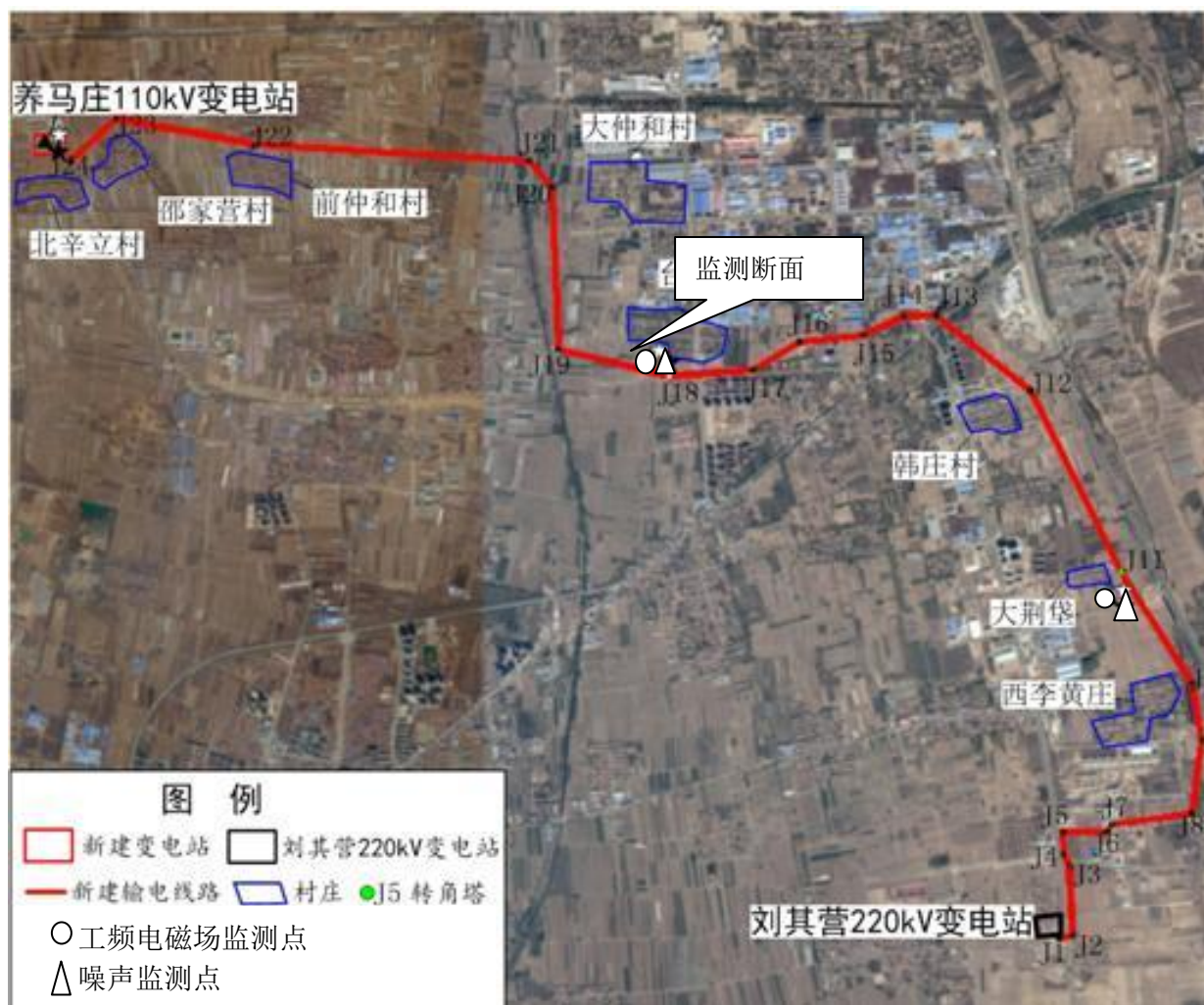
图 2 养马庄 110kV 输变电工程走向及监测布点监测示意图
