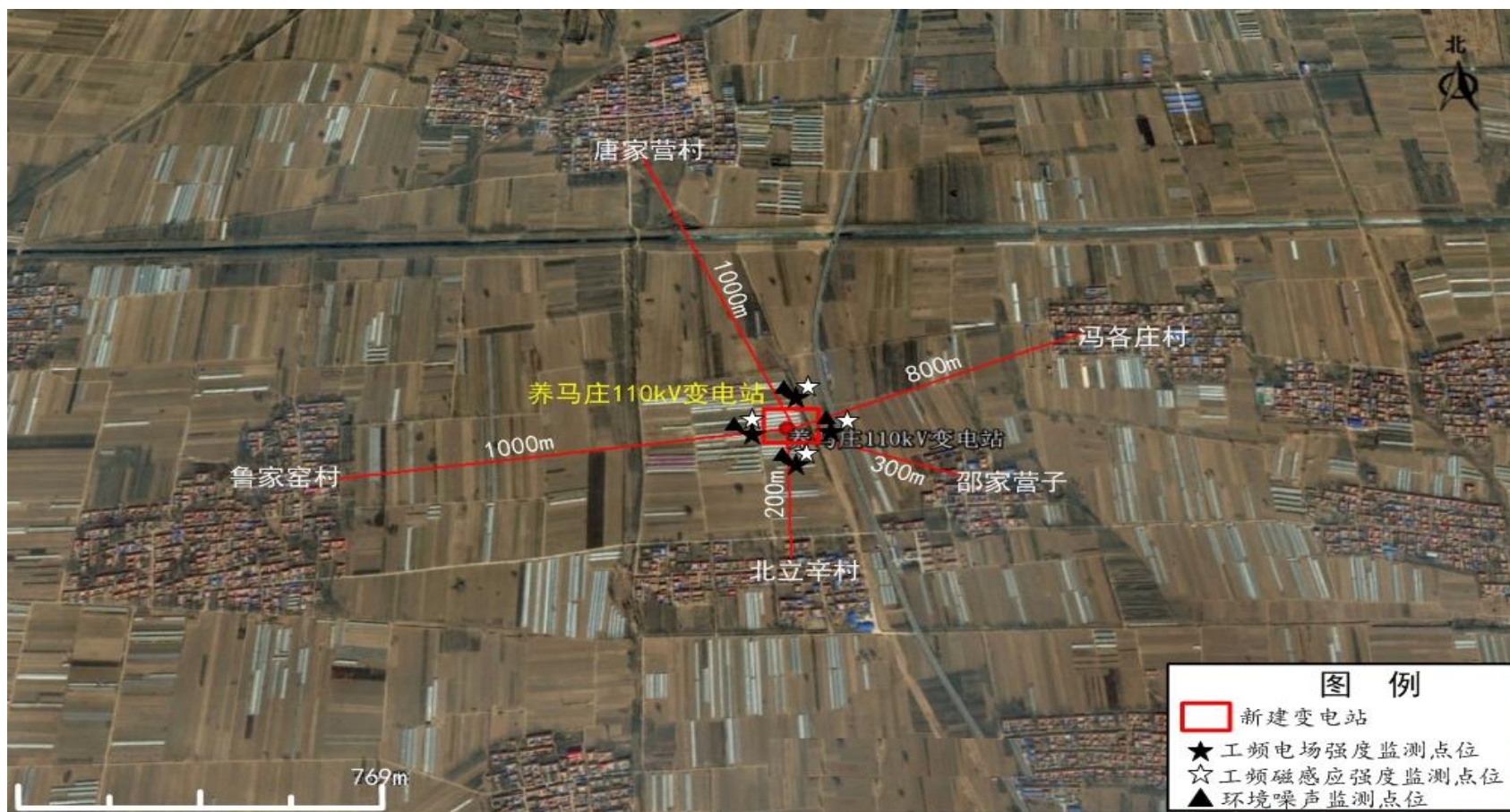
附图2 养马庄110kV变电站周围环境及验收检测布点图
