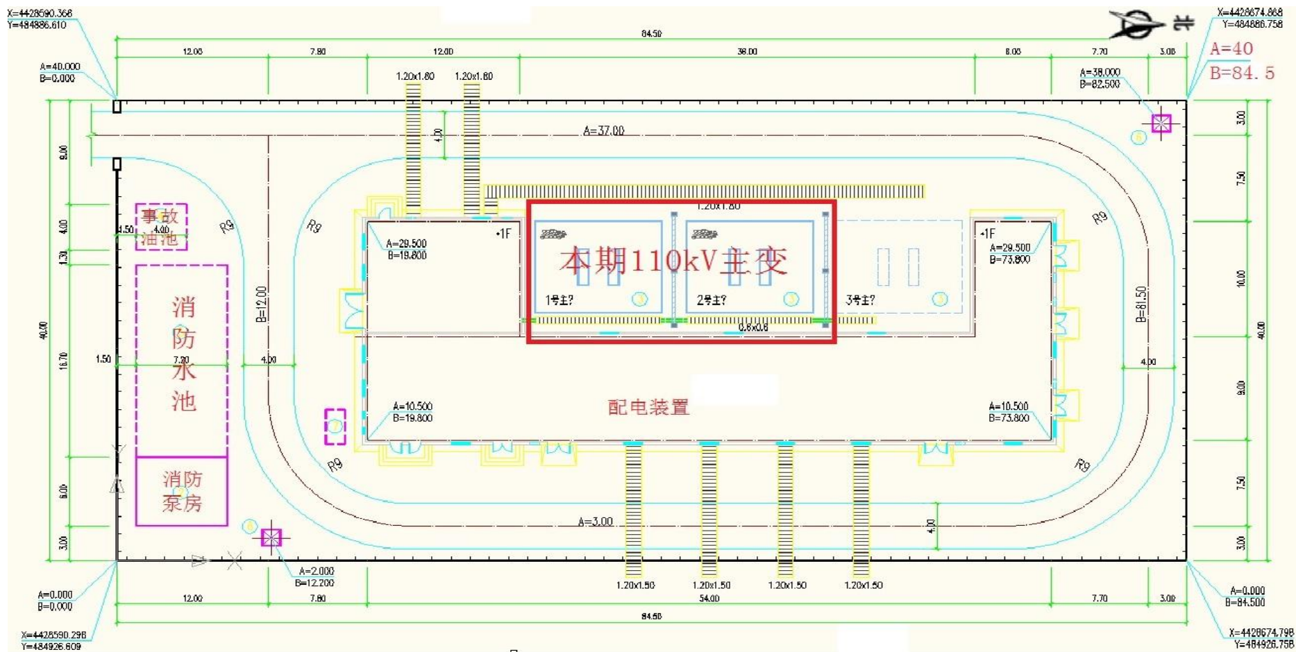
附图3 盛家屯110kV变电站电气平面布置示意图
