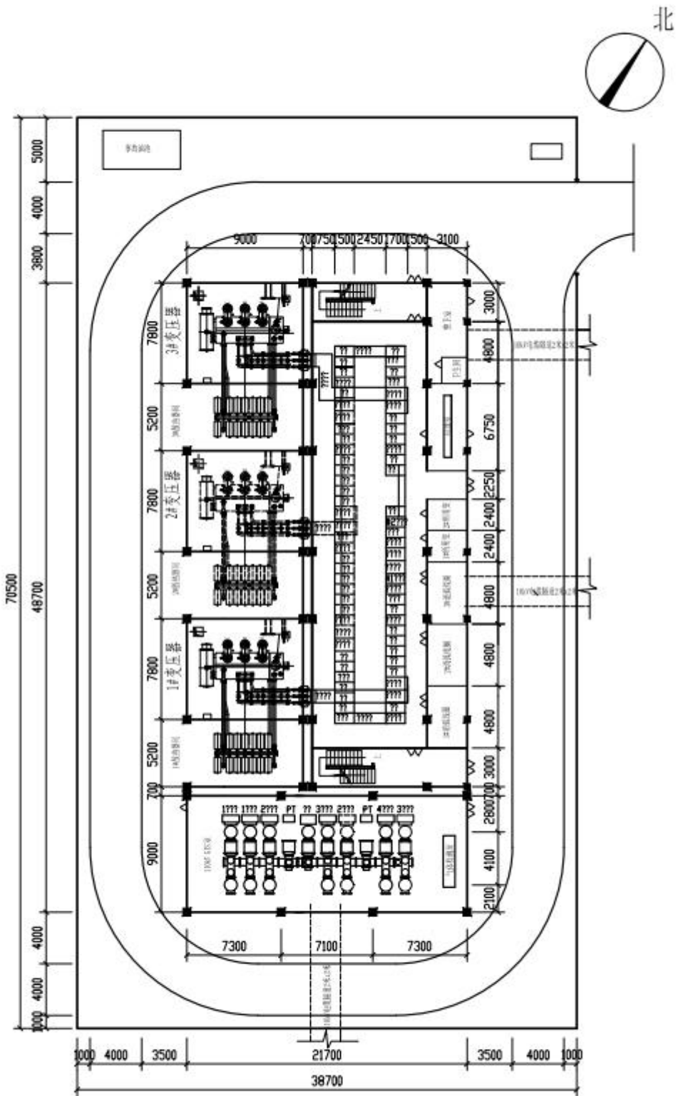
附图 3 唐山惠丰湖 110kV 变电站电气平面布置图
