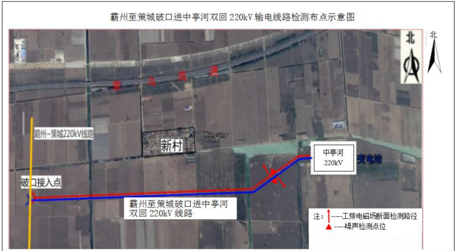
附图 4 中亭河 220kV 输变电工程新建线路路径及检测布点示意图
