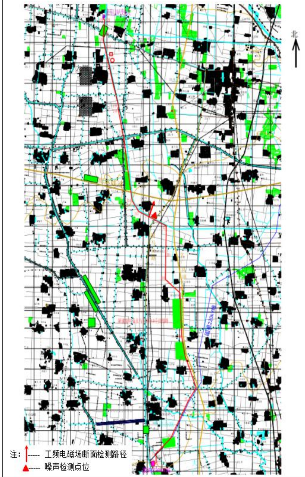
附图 4 北马 110kV 输变电工程新建线路路径
