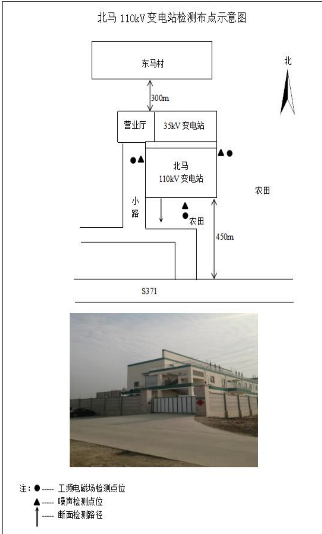
附图 2 北马 110kV 变电站监测布点示意图
